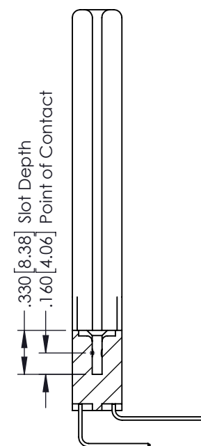
SECTION A-A
