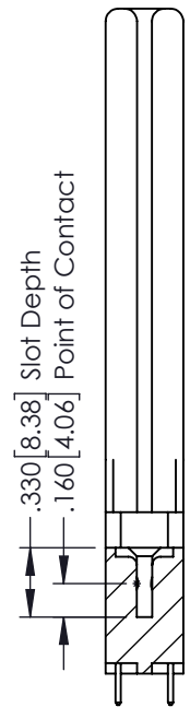
SECTION A-A
