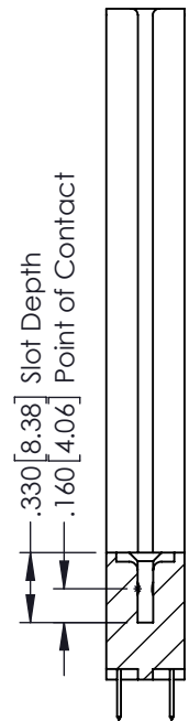
SECTION A-A
