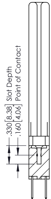
SECTION A-A
