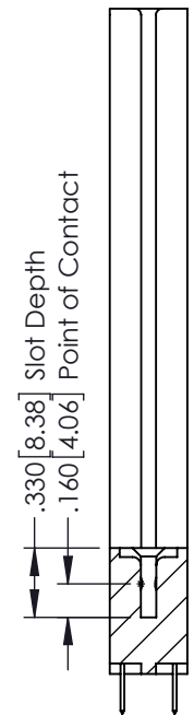
SECTION A-A
