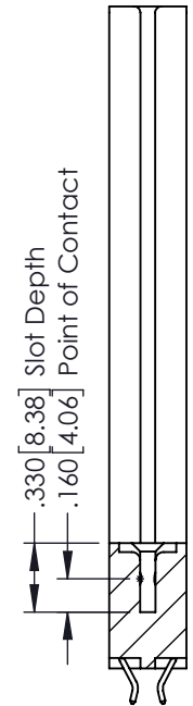
SECTION A-A
