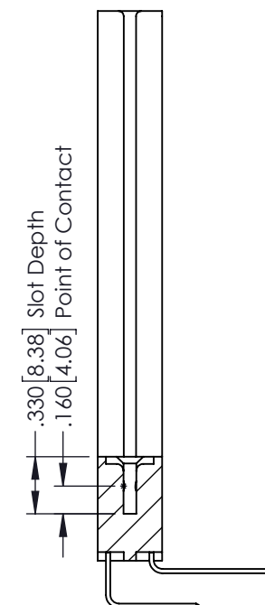
SECTION A-A
