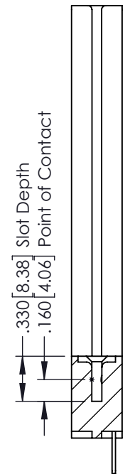
SECTION A-A
