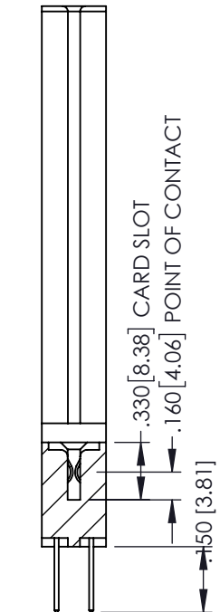
SECTION A-A
