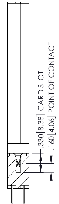
SECTION A-A
