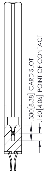
SECTION A-A
