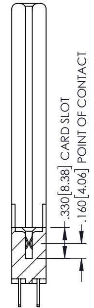
SECTION A-A
