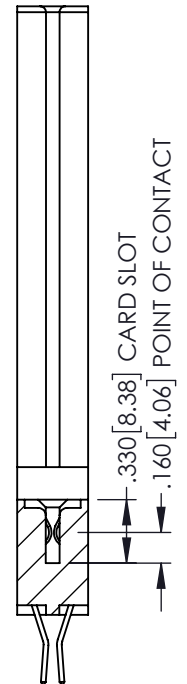
SECTION A-A
