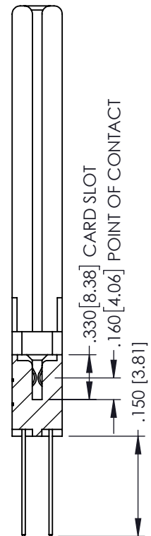
SECTION A-A
