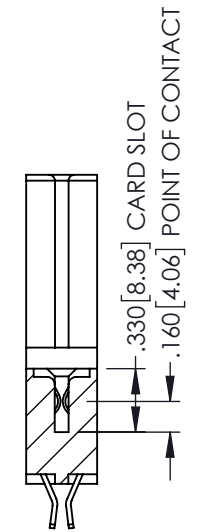
SECTION A-A
