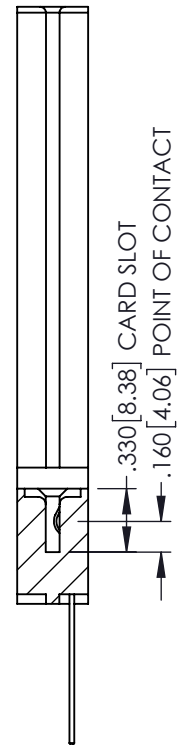
SECTION A-A
