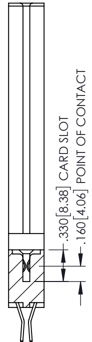
SECTION A-A
